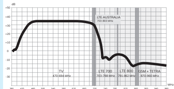
Courbe de gain
