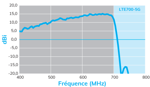
Courbe de gain
