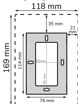
Dimension du moniteur et du support
